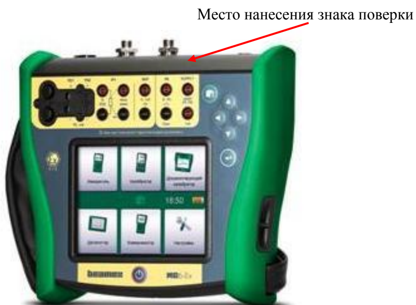
Рисунок 2 – Общий вид калибратора BEAMEX MC6-Ex (-R) с указанием места нанесения знака поверки
